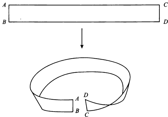
图 1.11 Möbius 带
