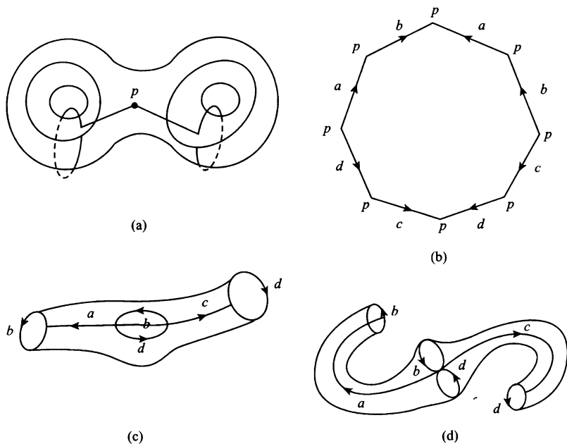
图 7.9 \Sigma_2 的典范表示
