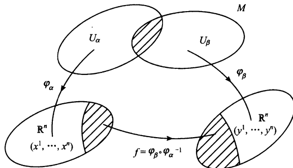
图 1.4 流形 M 的两个有交叠的坐标卡
