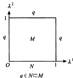
(7.31) 图 7.13 M 中相对 N 以 q 点为基点的 2 环路示意图
