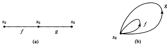
图 7.4 h = f \circ g 的示意图, (a) 为源图, (b) 为像图
