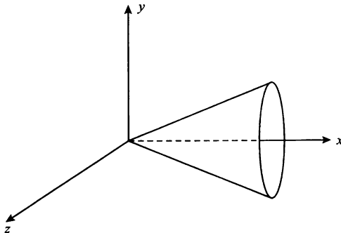
图 1.3 E^3 中半锥面
