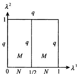
图 7.14 两个相对 2 环路相乘的示意图
