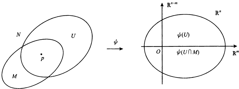
图 2.3 子流形 M 的正则坐标卡
