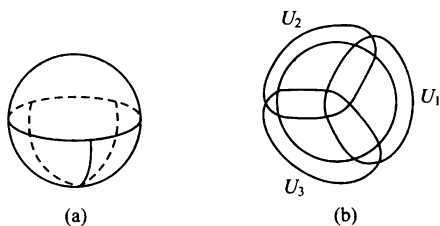
图 9.4 2 维球面 S^2 的好覆盖
