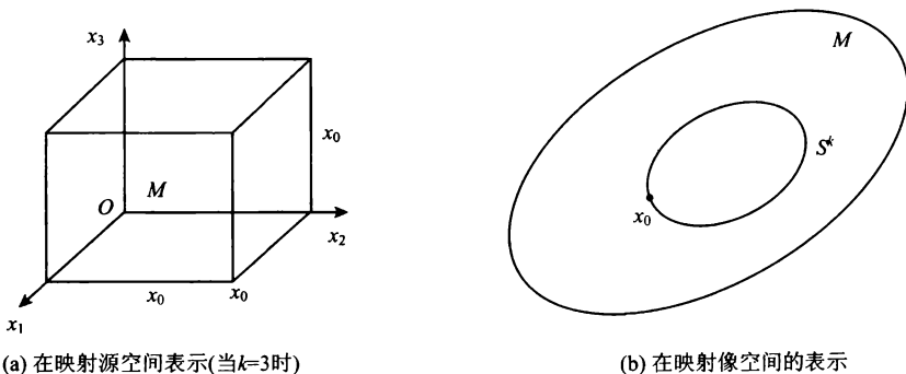
图 7.10 k 维环路映射示意图
