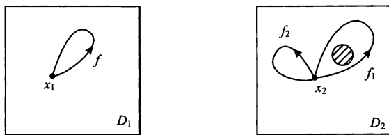
图 7.3 环路同伦等价类示意图
