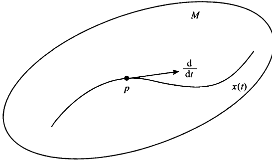
图 1.9 利用曲线 x(t) 选出过 p 点确定方向
