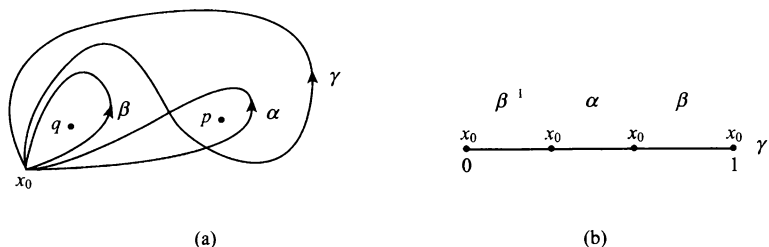
图 7.7 具有两个洞的二维开区间上环路示意图
