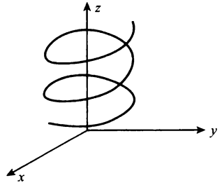
图 2.2 \mathbb{R}^3 中螺旋线
