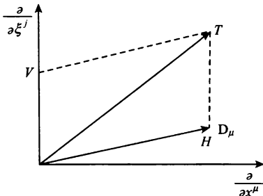
图 14.1 丛 E 的切丛 T(E) 分解示意图
