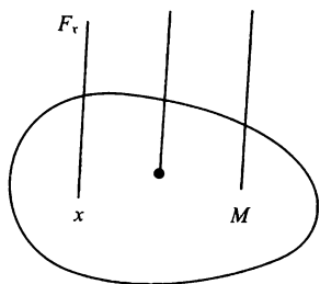
图 13.1 向量丛 E 示意图
