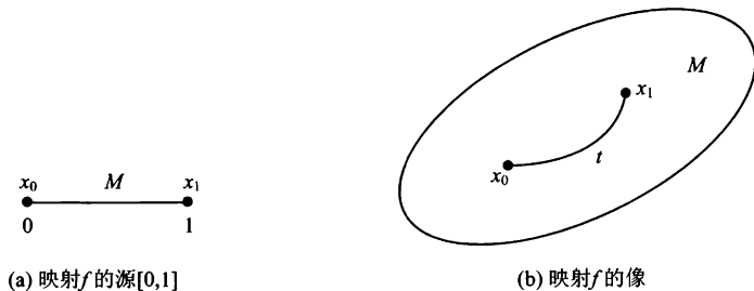
图 7.2 路径的示意图
