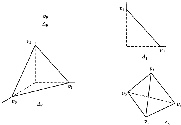
图 7.16 最初的几个标准 k 单形
