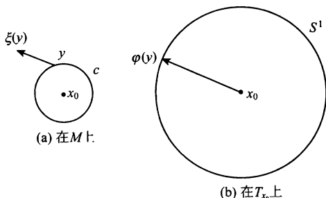
图 18.1 Gauss 映射示意图
