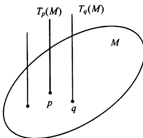
图 1.10 切丛示意图
