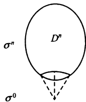
图 9.1 单点 \sigma^0 与 例 9.2 2 维定向面(见图 7.9)
