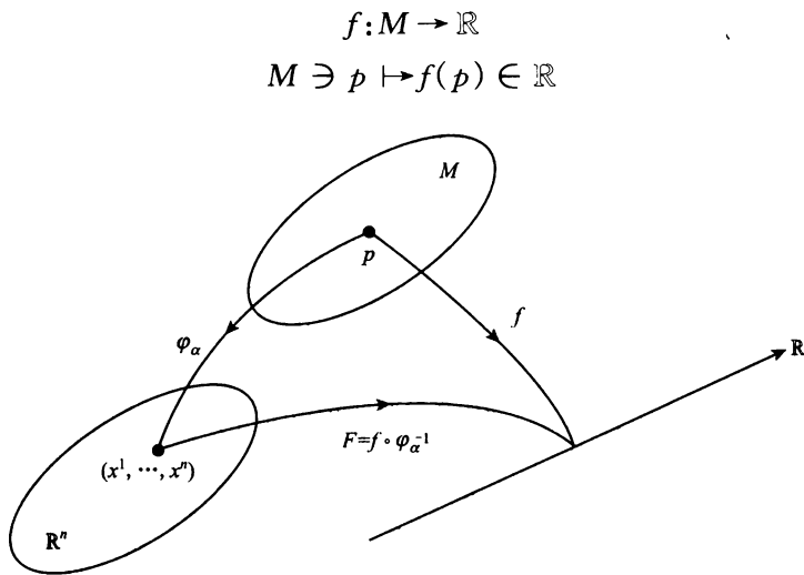
图 1.5 流形上的函数 f(p)
